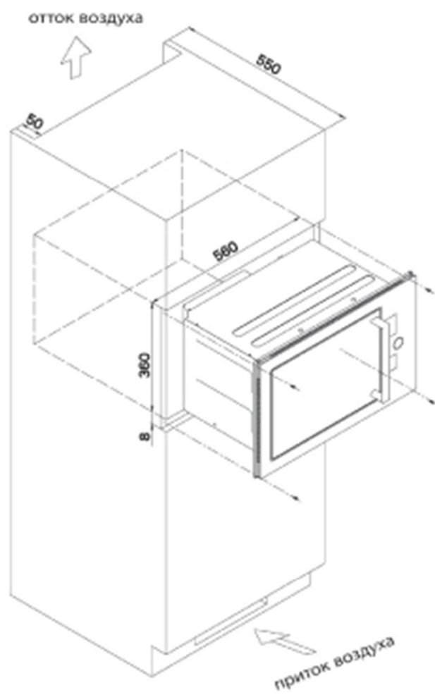
Схема установки
